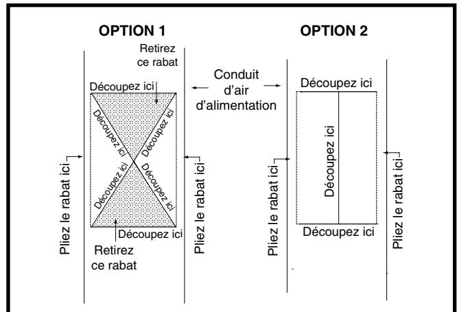
Figure 11. Ouvertures étroites de conduit d'air
