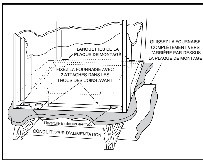
Figure 14. Fournaies de placard « A » et « B »
