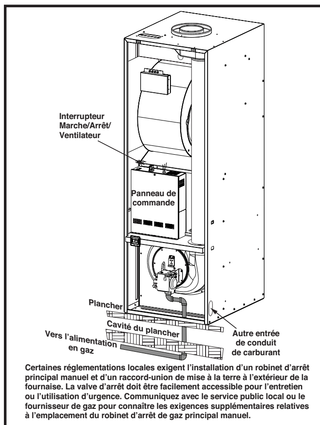
Figure 2. Composants de la fournaise au gaz MG1
