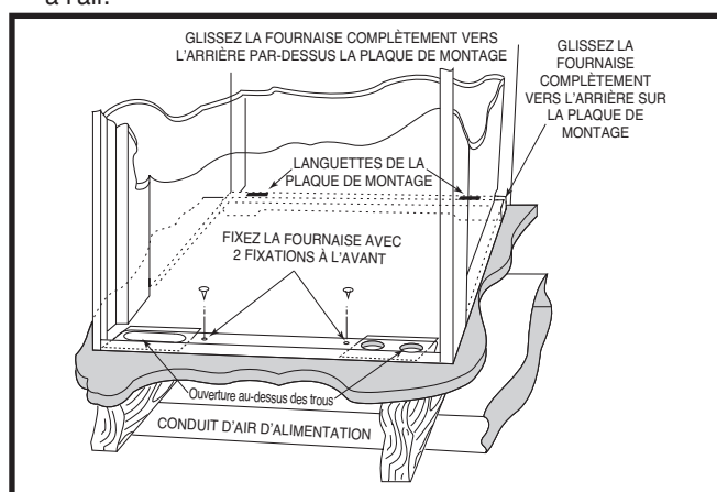
Figure 17. Fournaise de placard sur conduit d'air d'alimentation
