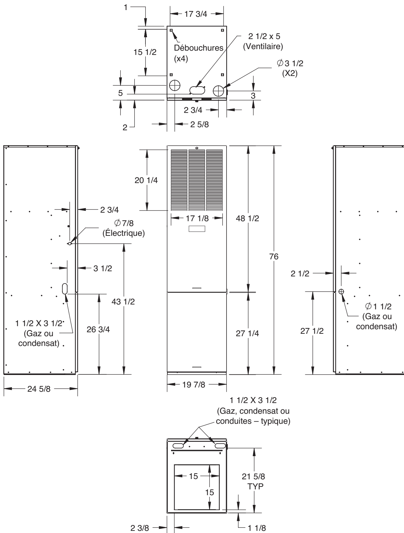
Figure 27. Armoires à reprise d'air avant (avec boîtier de serpentin) (armoires à reprise d'air avec le suffixe ACM)
