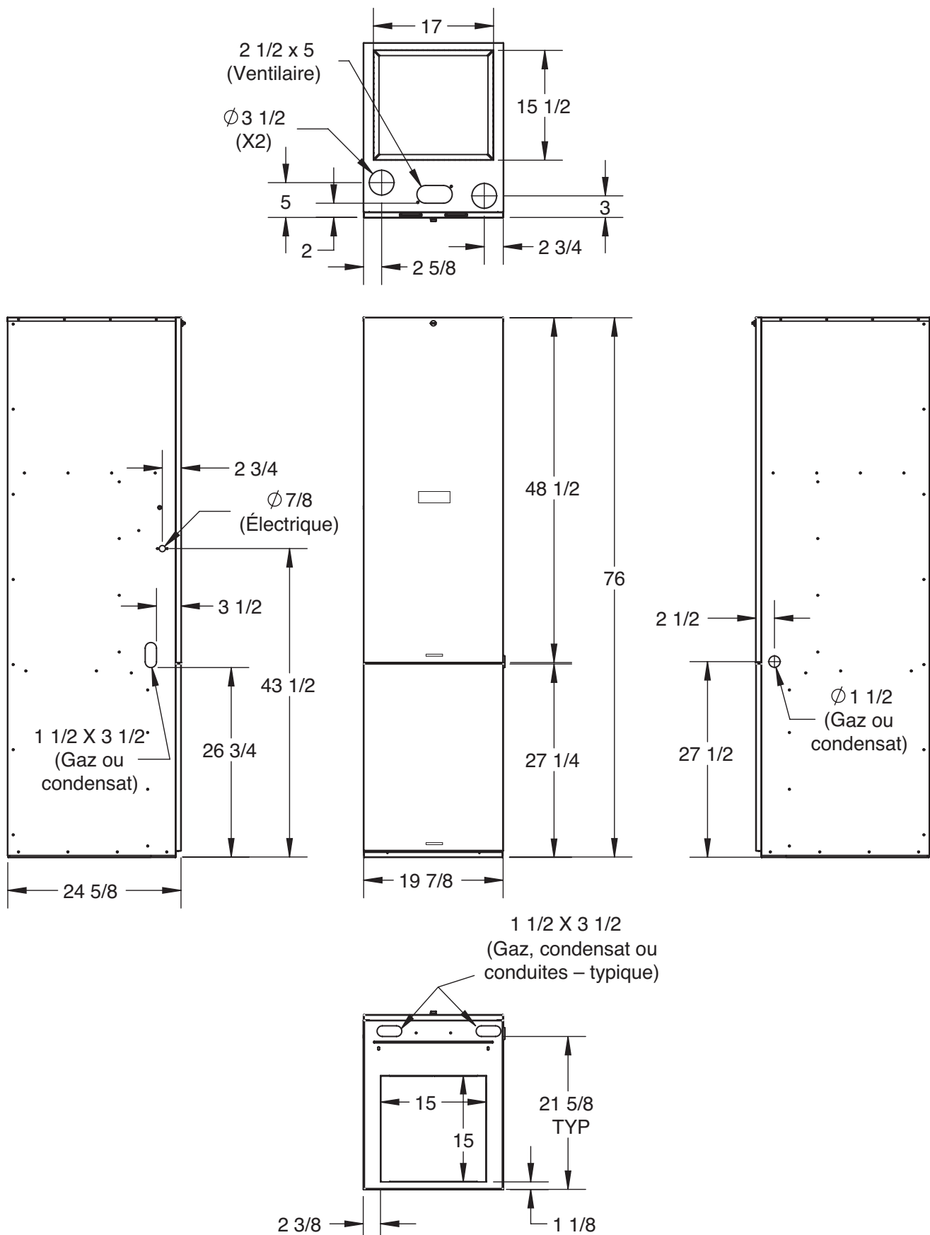
Figure 30. Armoires de reprise d'air par le haut (avec boîtier de serpentin) (armoires de reprise d'air avec le suffixe ACM)
