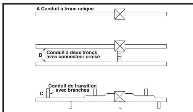
Figure 7. Systèmes de conduit d'alimentation typiques
