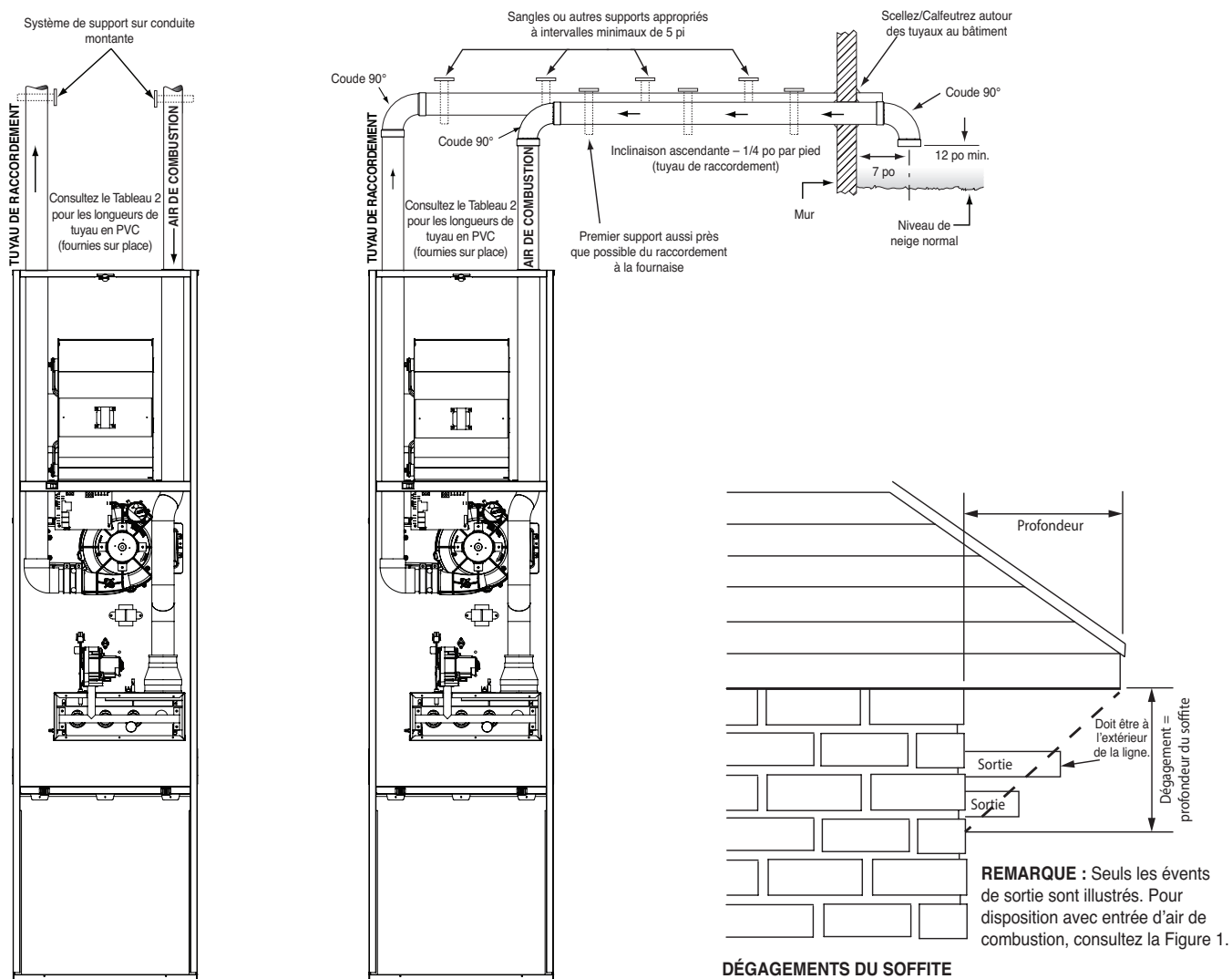
Figure 33. Évacuation horizontale/verticale et dégagements au soffite
