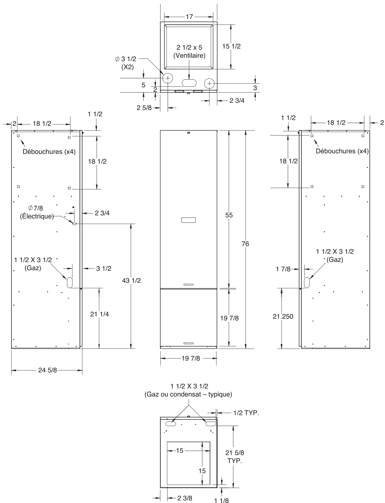
Figure 29. Armoires de reprise d'air par le haut (avec boîtier de serpentin) (armoires de reprise d'air avec le suffixe ABM)
