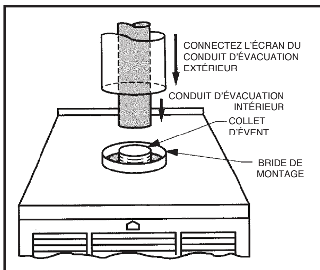
Figure 23. Branchement du tuyau d'air de combustion
