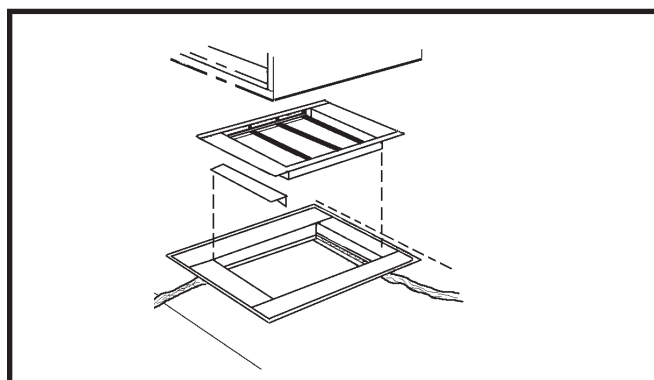
Figure 32. Sans registre de cavité à serpent
