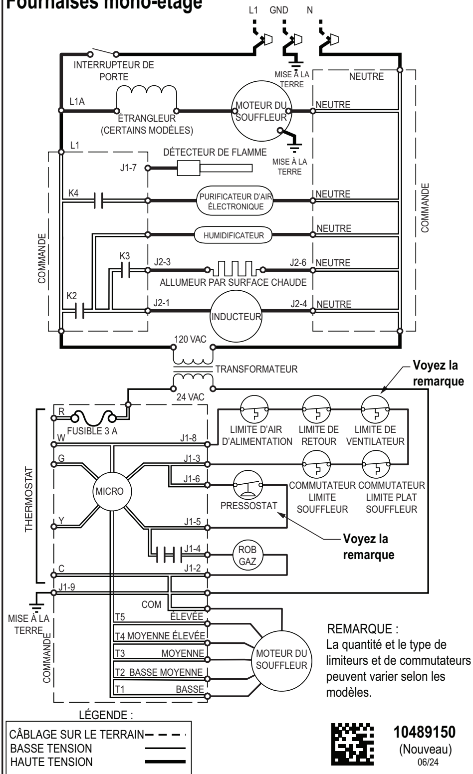
Figure 34. Schéma en échelle Nordyne Channel
