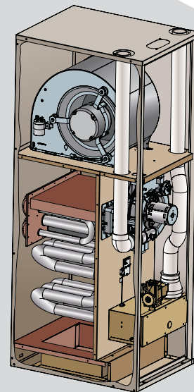
95.1% AFUE cutaway view shown
